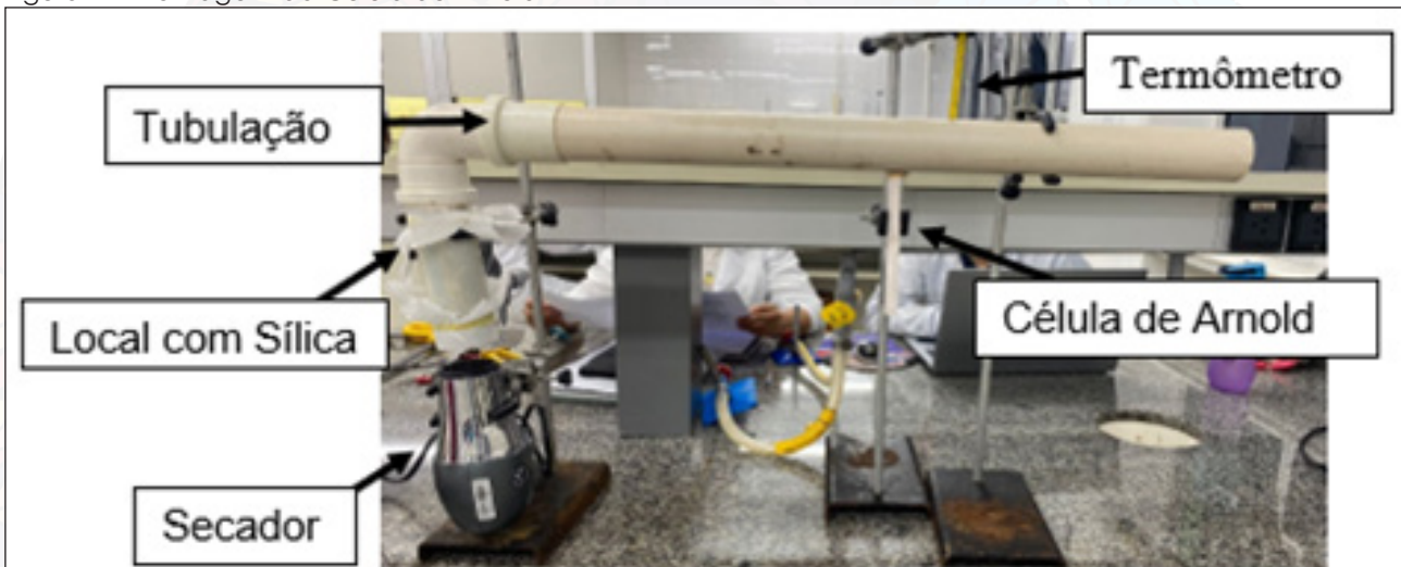
Figura 1 – Montagem da Célula de Arnold
