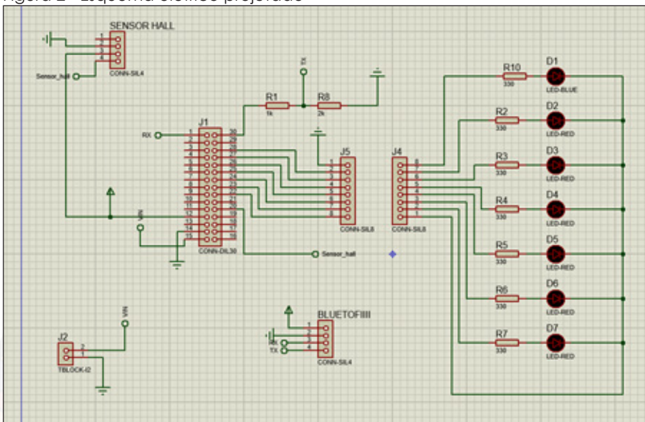
Figura 2 - Esquema elétrico projetado
